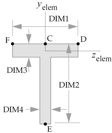
TYPE="T"
