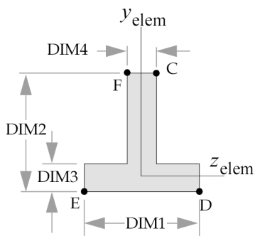
TYPE="T2"
