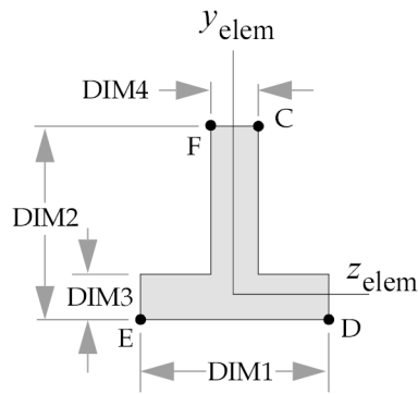
TYPE="T2"
