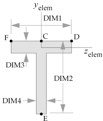
TYPE="T"
