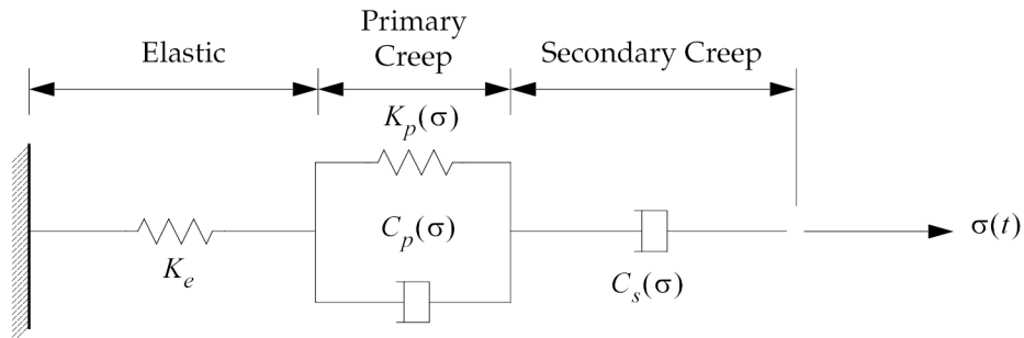
Figure 13-25. CREEP Parameter Idealization
